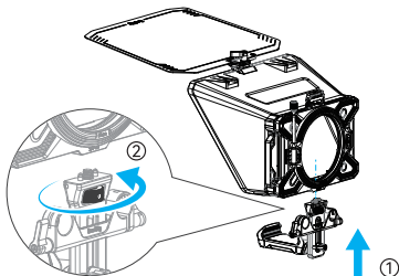
Install the Clamp-on back 95mm 安装 95mm背板
